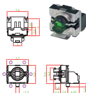
TC009L-N11ABAX□□□□
