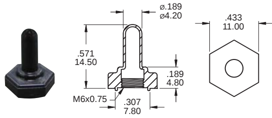
PU2-ET-102
