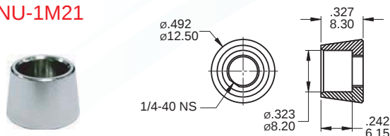
MNU-1M21
