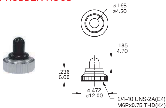
E4-RUBBER-HOOD K4-RUBBER-HOOD
