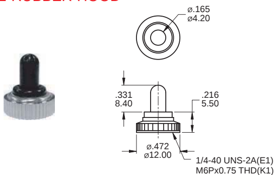
E1-RUBBER-HOOD K1-RUBBER-HOOD
