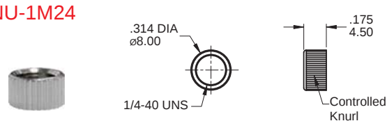
MNU-1M24
